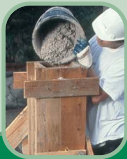
Coulage d'un poteau en béton
